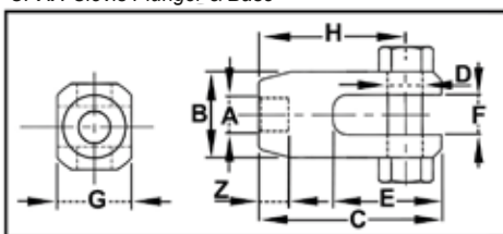
CPXX-Clevis Plunger &amp; Base
