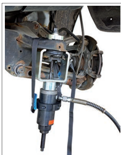
Silentbloc overview
