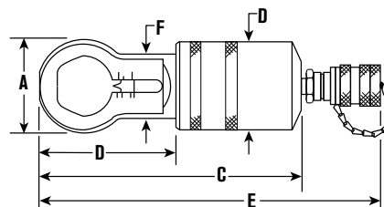
HNS150 & HNS225
